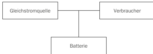
Abb. 6-2: Bereitschaftsparallelbetrieb
